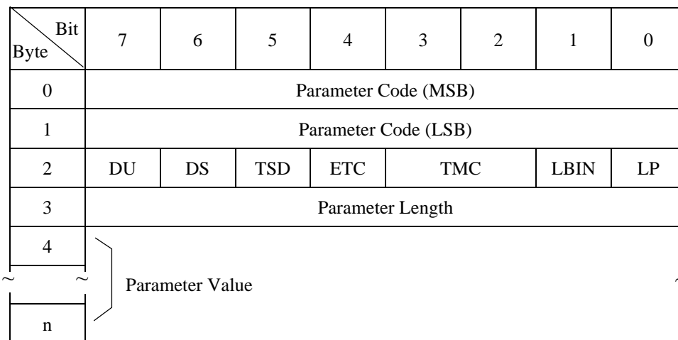
Figure 3.14 LOG SELECT command: log parameter
